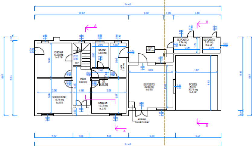
PIANTA PIANO TERRA STATO REALIZZATO
