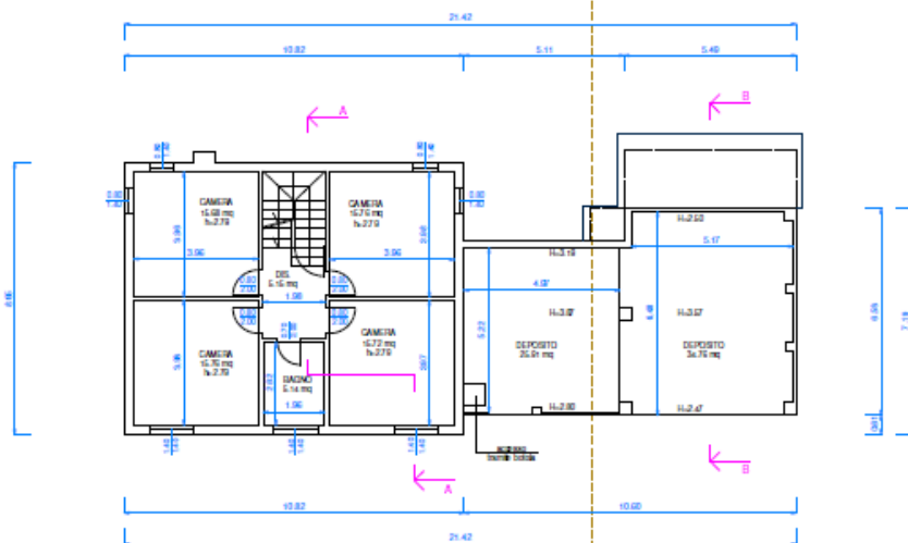
PIANTA PIANO PRIMO STATO REALIZZATO
