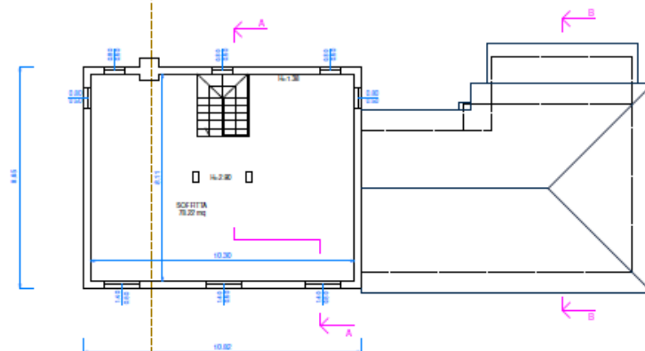
PIANTA PIANO SECONDO STATO REALIZZATO
